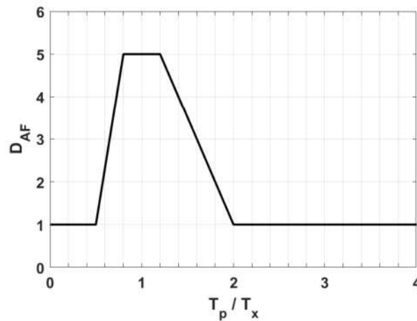
그림 18.2-1 비구조요소의 동적증폭계수 D_{AF}
